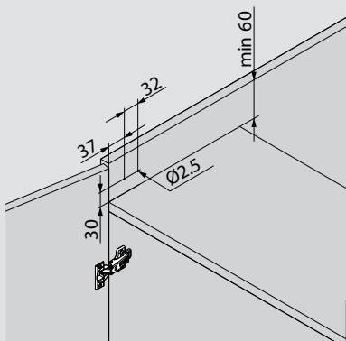
Vŕtanie pre montážnu podložku
