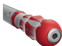
Griff-Stirnseite Verstellwerkzeug und Verlängerung mit Bitaufnahme 1/4"
